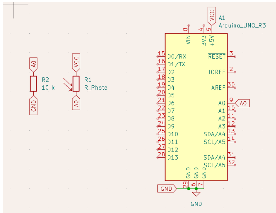
図 21 楽器デバイスの受光部の回路図
