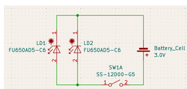
図 20 レーザー回路図
